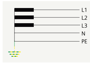
TN-S Sistem
