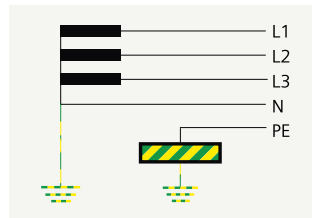
TT Sistem
